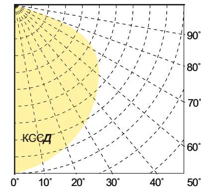
КРИВАЯ СИЛЫ СВЕТА
