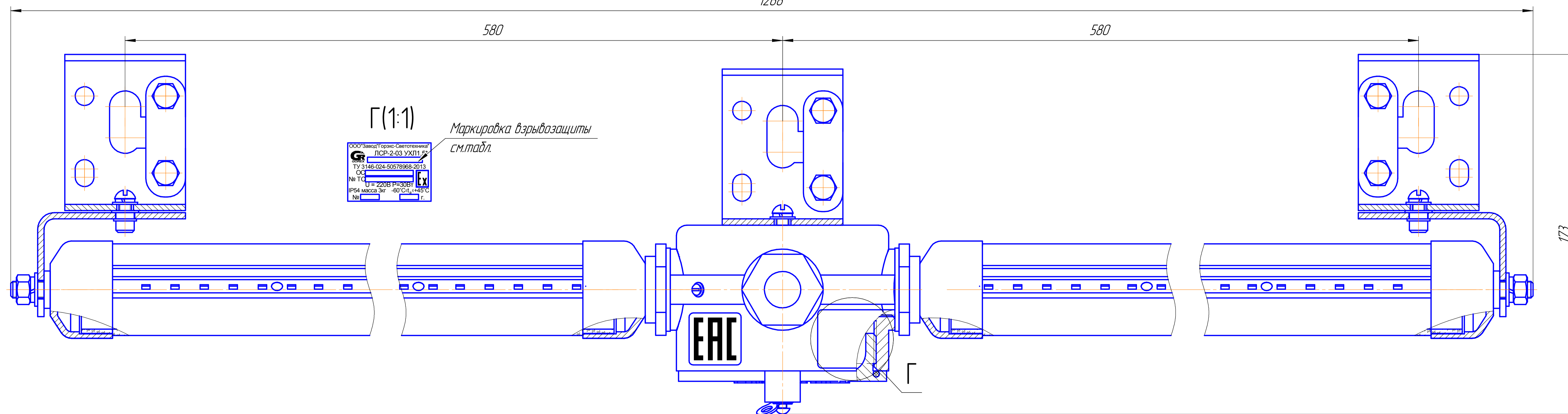
Рисунок 1-Общий вид и чертёж средств взрывозащиты Светильников взрывозащищенных рудничных ЛСР-1-03 и ЛСР-2-03
